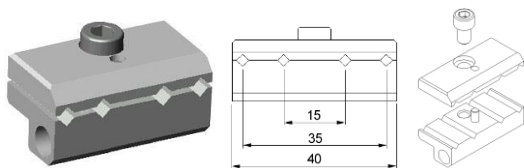
Zacisk grotowkrętów L=40mm
